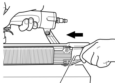
Alimenteur d'agrafes
