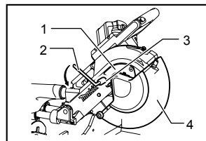
1. Couvercle central 2. Clé à douille 3. Boulon hexagonal 4. Protecteur de lame
