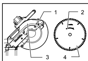
1. Flèche 2. Flèche 3. Boîtier de la lame 4. Lame
