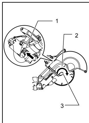
1. Verrouillage de l'arbre 2. Boîtier de la lame 3. Boulon hexagonal
