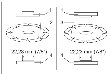
► 1. Contratuerca 2. Rueda de diamante (con un grosor menor de 4 mm (5/32")) 3. Rueda de diamante (con un grosor de 4 mm (5/32") o mayor) 4. Brida interior
