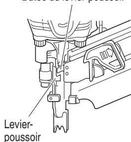
Butée du levier-poussoir
