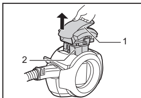
1. Palanca de liberación del compartimento 2. Montaje del compartimento para polvo
