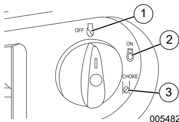
Figura 2-5. Interruptor (ejemplo)
