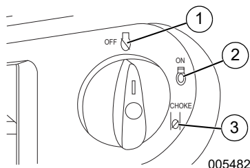
Figure 2-5. Commutateur (exemple)
