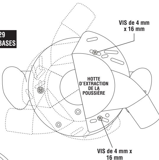
Hotte d'extraction de la poussière
