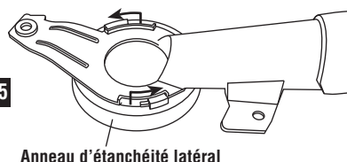
FIG. 26 Vis à serrage à main de 4 mm Anneau d'étanchéité latéral Hotte d'extraction de la poussière (Accessoire en option)
