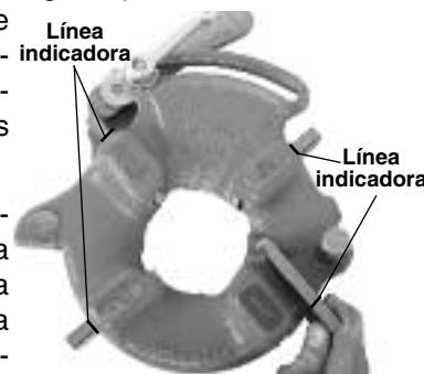
Figura 8 – Inserción de terrajas hacia el final de la ranura (Figura 8).
