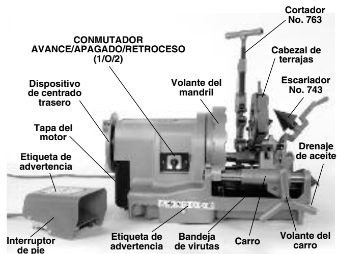
Figura 2 – Roscadora 1233
