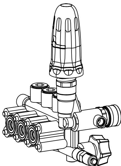
TC3-K2 TC3-13X13.0 MANIFLOD KIT
