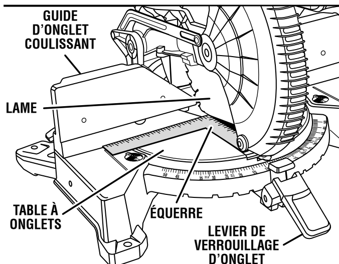
VUE DE LA LAME PAS D'ÉQUERRE AVEC LE GUIDE, DES RÉGLAGES SONT NÉCESSAIRES Fig. 17
