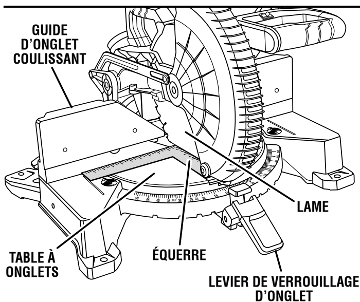
VUE DE LA LAME D'ÉQUERRE AVEC LE GUIDE Fig. 16
