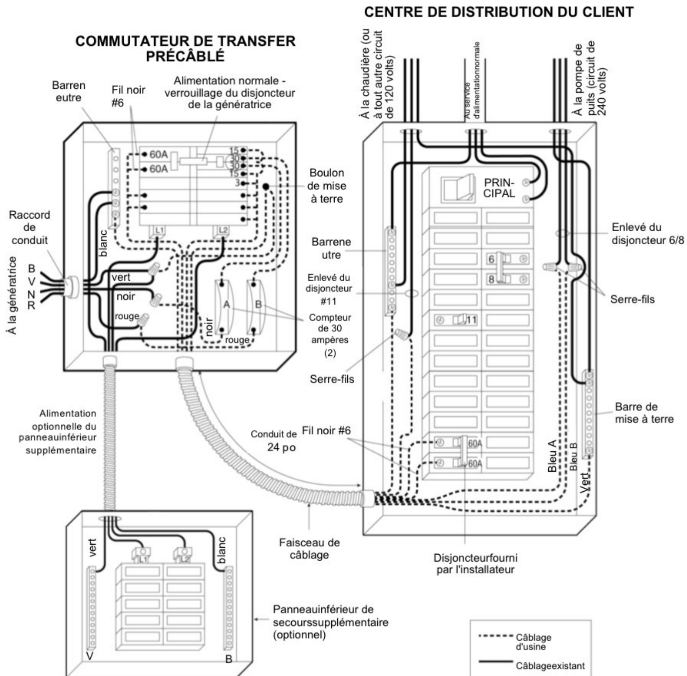
Figure 2: DIAGRAMME DE CÂBLAGE
