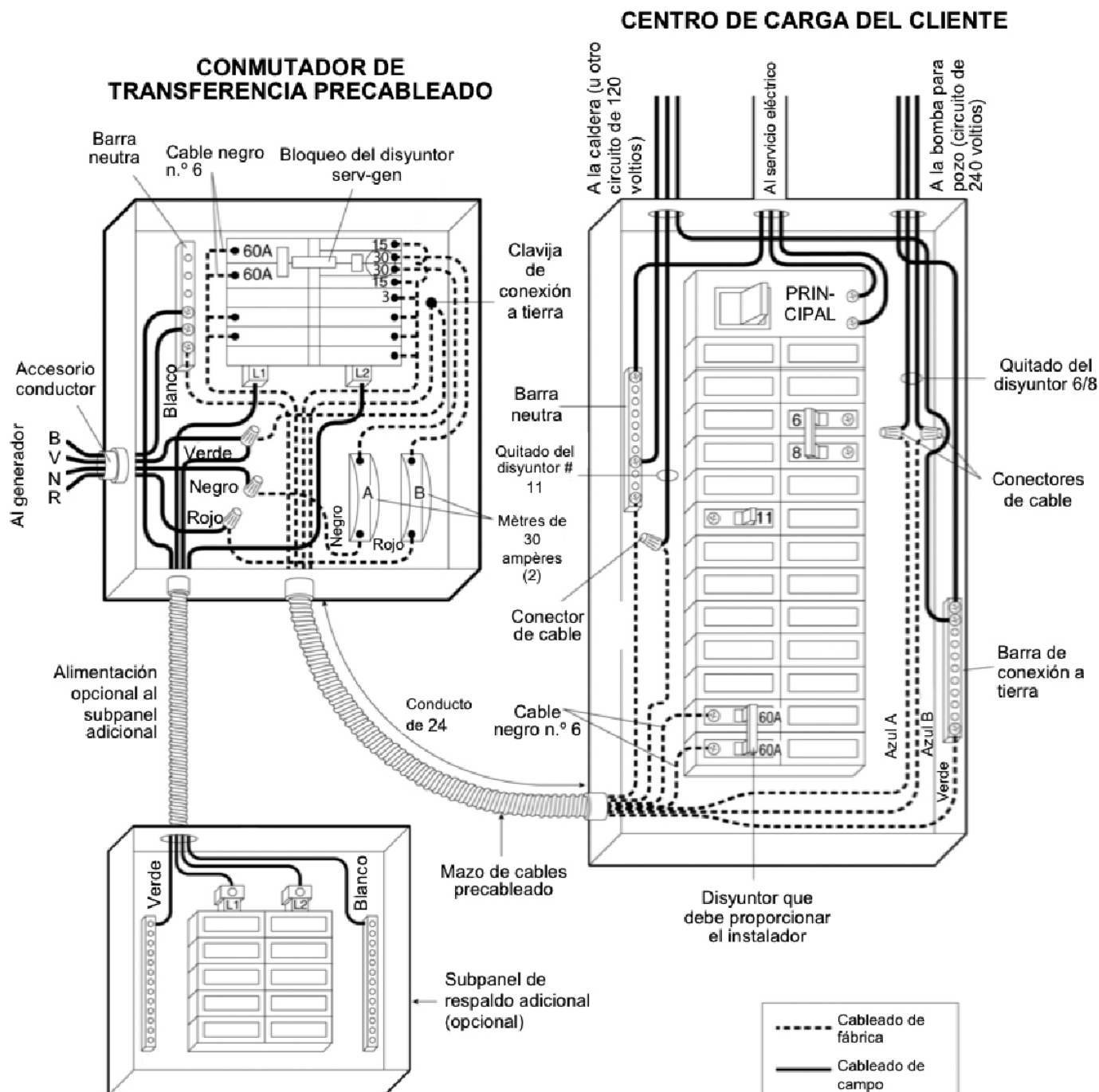
Figura 2: DIAGRAMA DE CABLEADO
