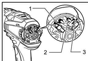
1. Bras 2. Ressort 3. Partie encastrée
