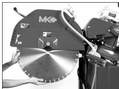
(D) Install the Diamond Blade onto the Blade Shaft.
